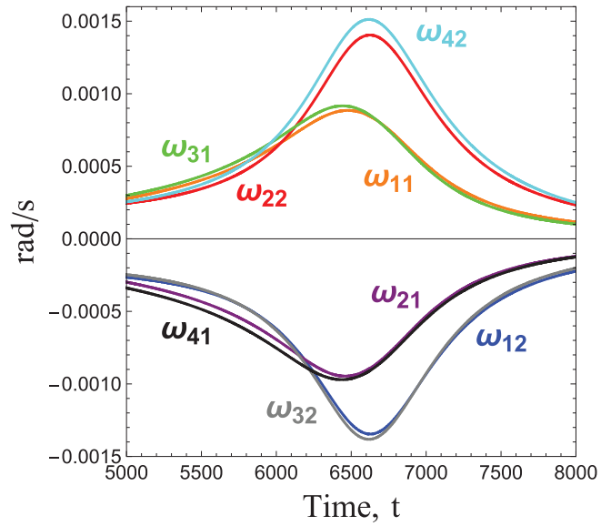
(d) Revolute link angular velocities
